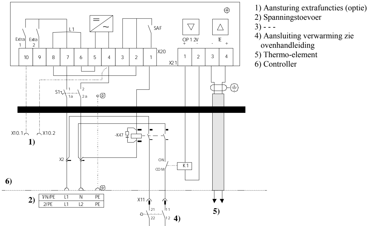
Fig. 34: Vervanging voor S-controllers
