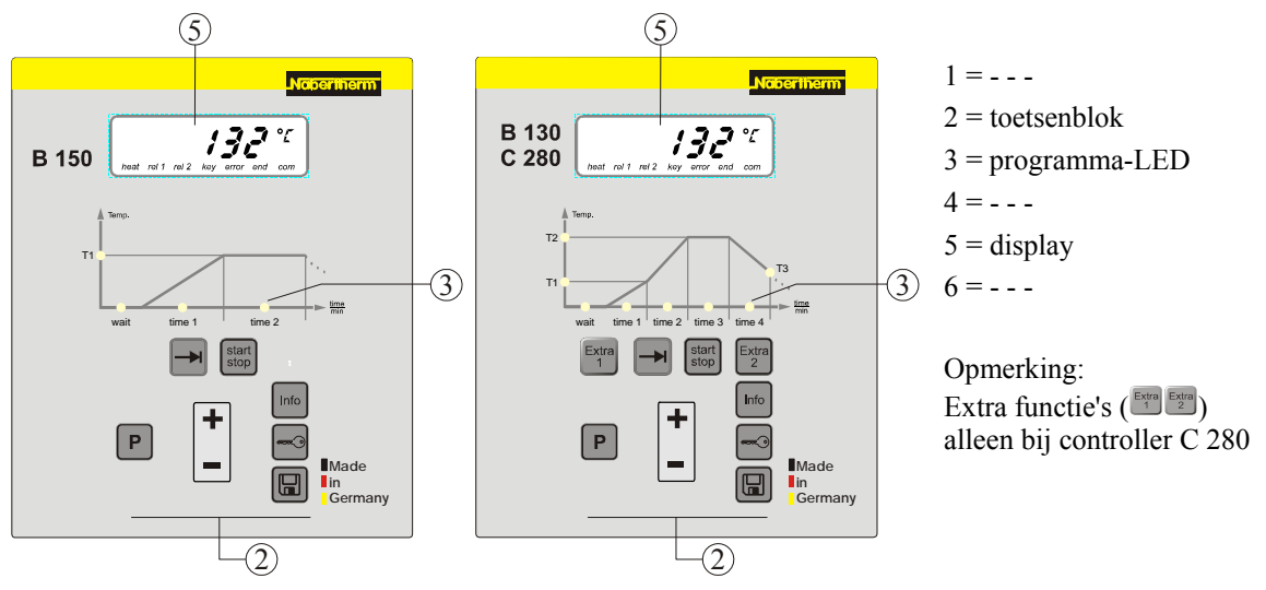
Afb. 1: Bedieningsveld B 150/B 130/C 280
