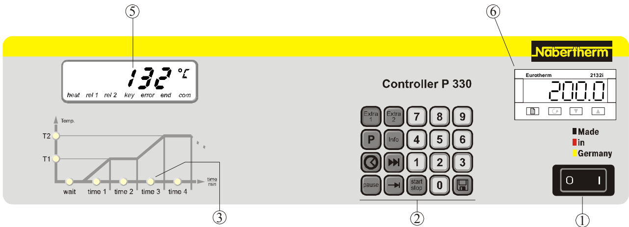
Fig. 2: Bedieningsveld P 330
