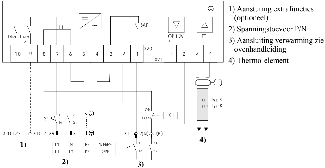
Fig. 28: Ovens tot 3,6 kW
