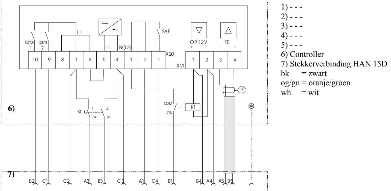
Fig. 35: Vervanging C-controller
