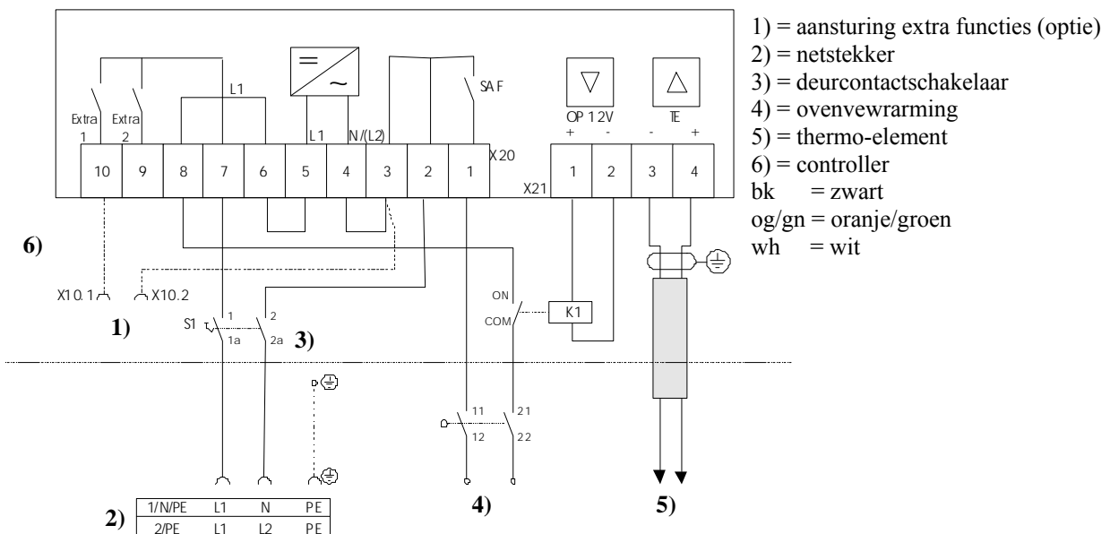
Fig. 33: Vervanging voor oude S-controllers tot 3,6 kW
