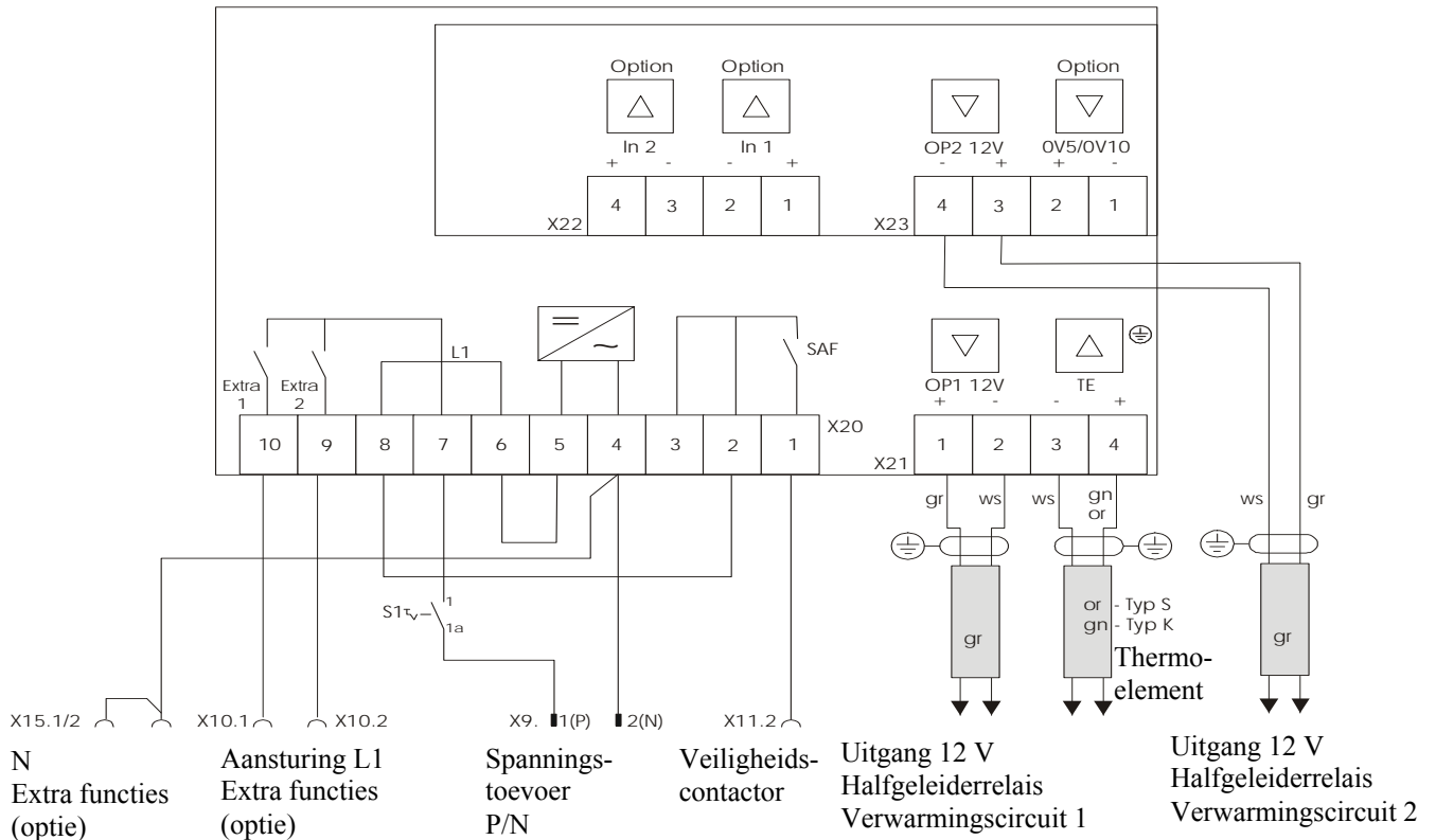
Fig. 32: Ovens > 3,6 kW met 2 verwarmingscircuits – P 310
