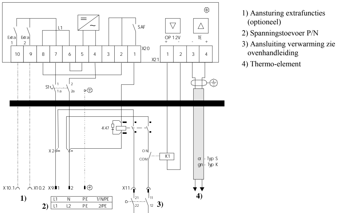
Fig. 29: Ovens tot 3,6 kW
