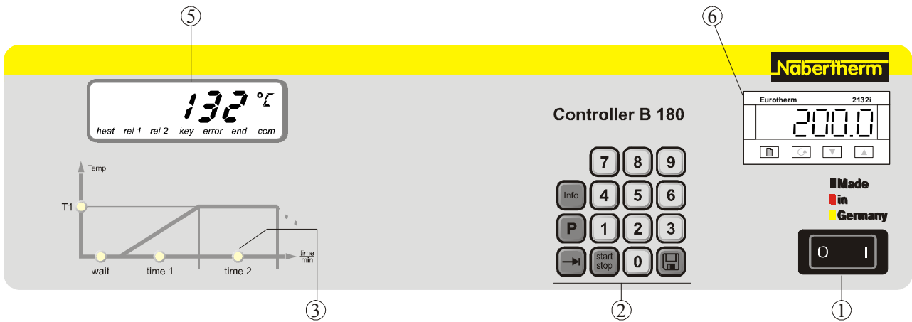
Fig. 1: Bedieningsveld B 180
